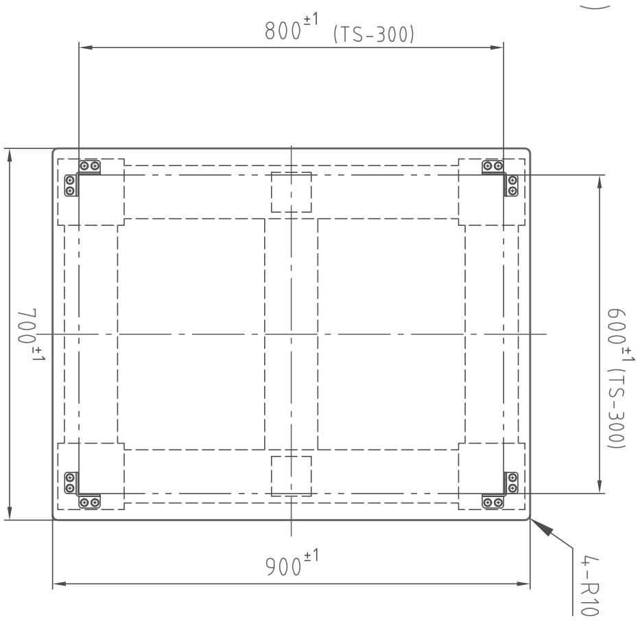
(平面图)
