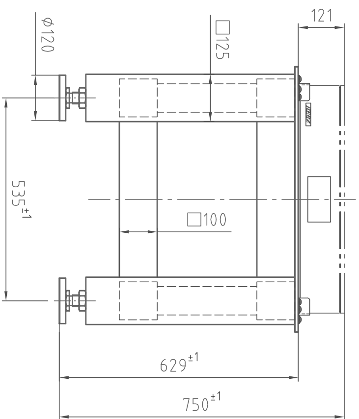
(正面图)
