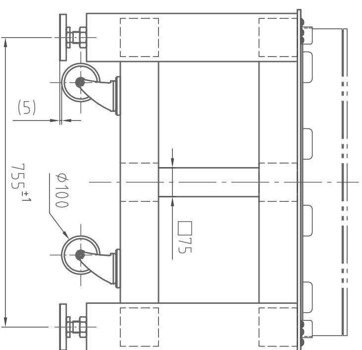
(右侧面图)
