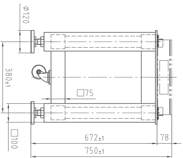
(正面图)
