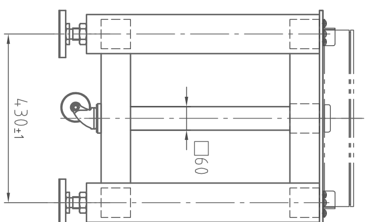
(右侧面图)
