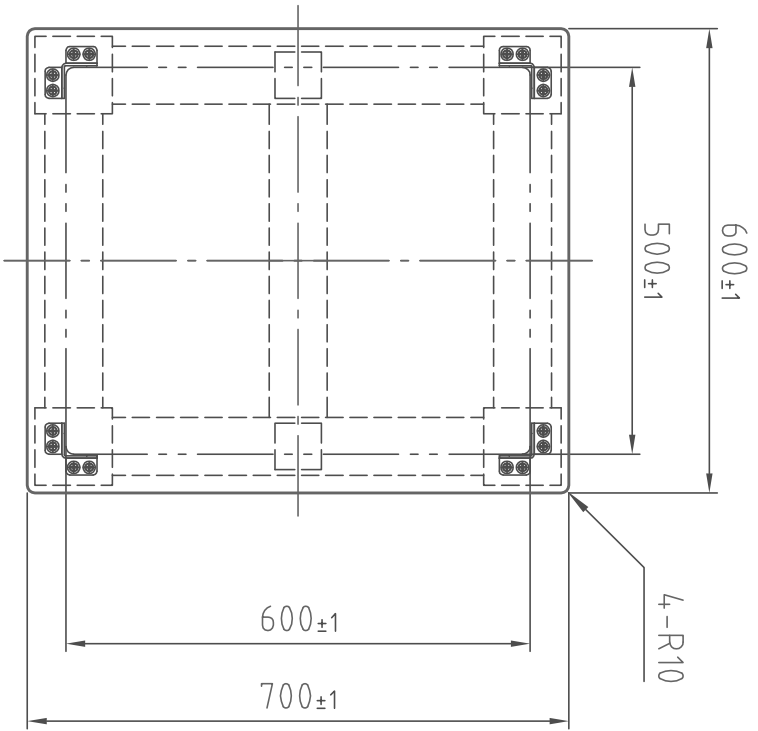
(平面图)
