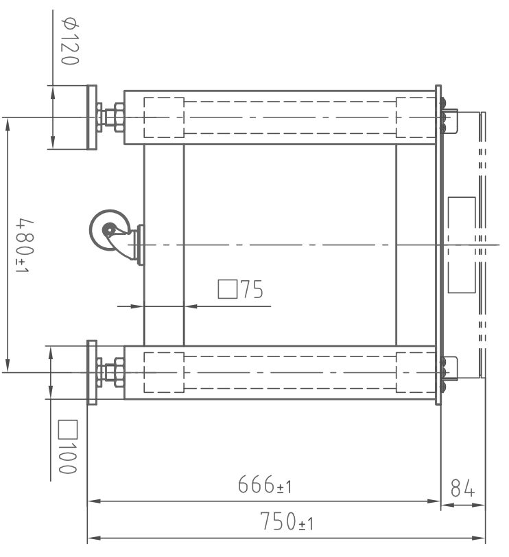
(正面图)
