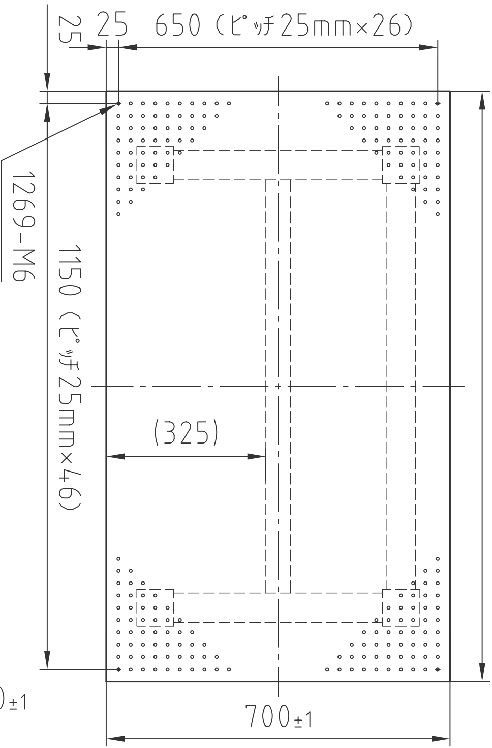
(平面図)
