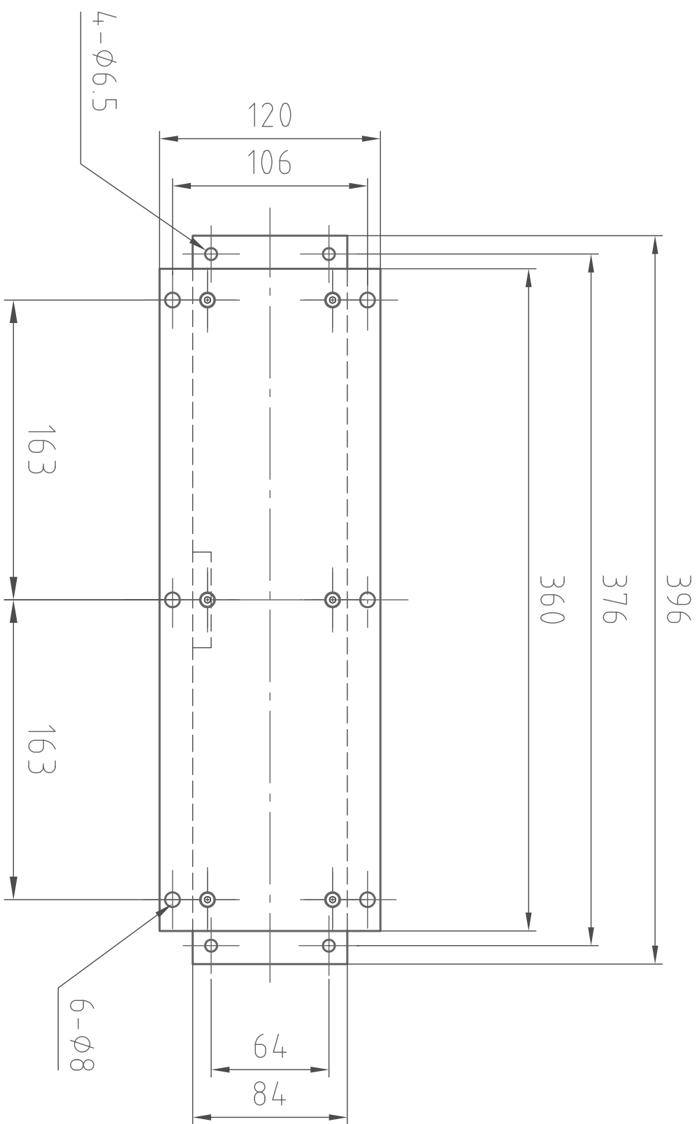
(正面図)
