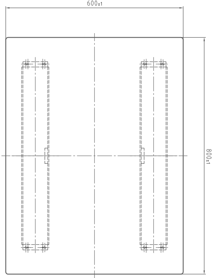
(平面図)
