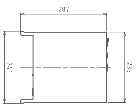
(平面図)
