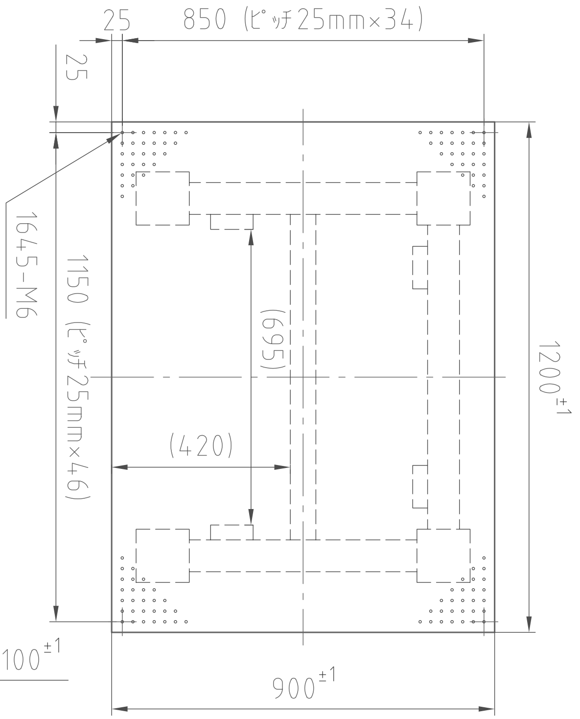
(平面図)
