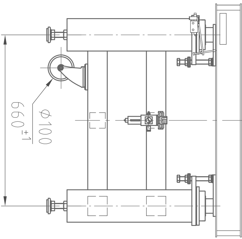
(右側面図)
