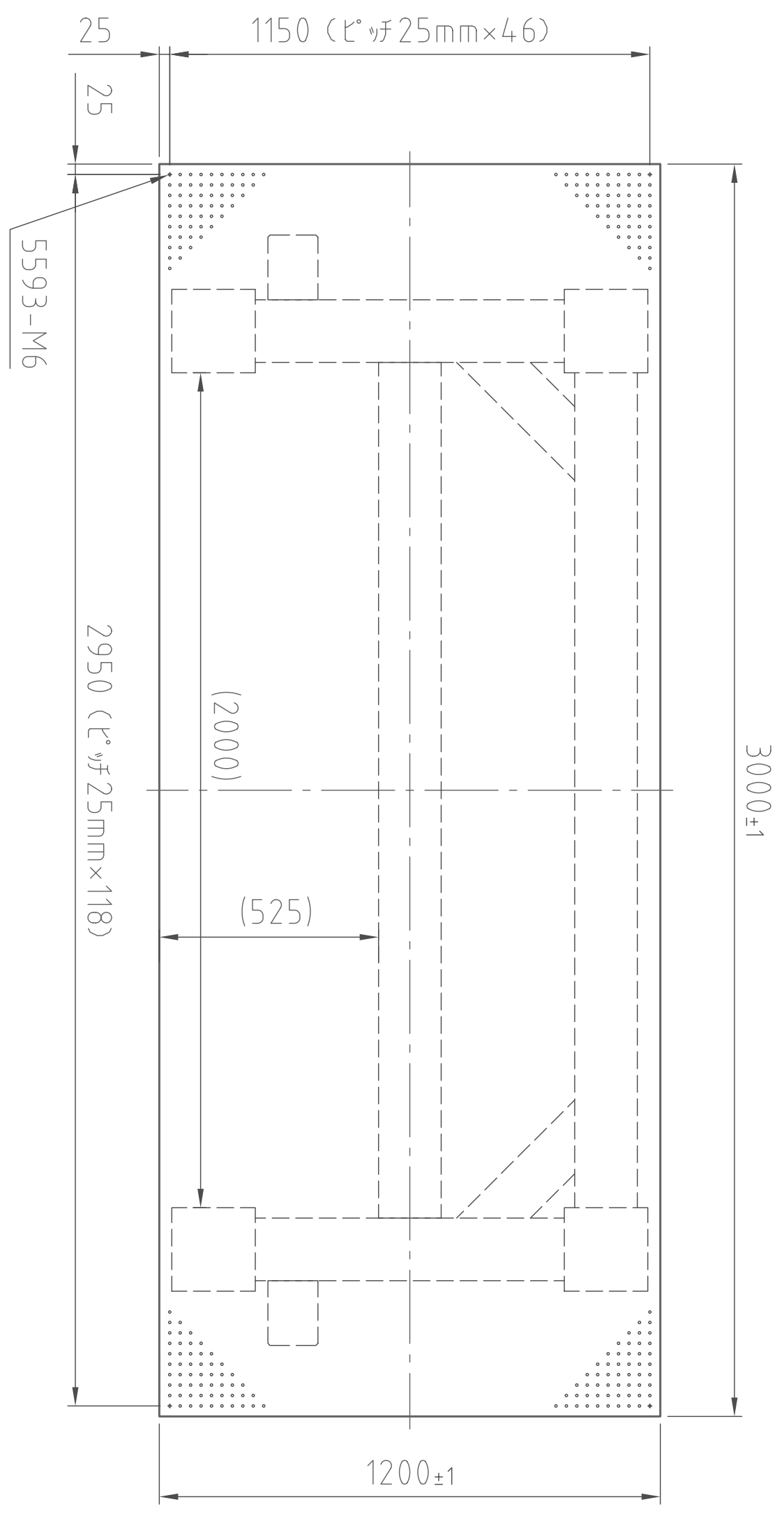
(平面図)
