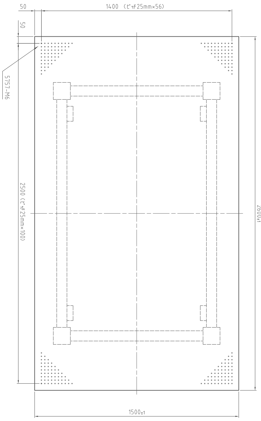
(平面图)
