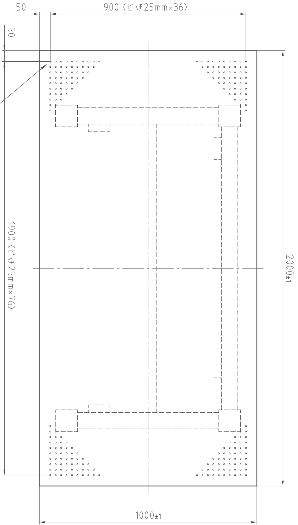
(平面图)
