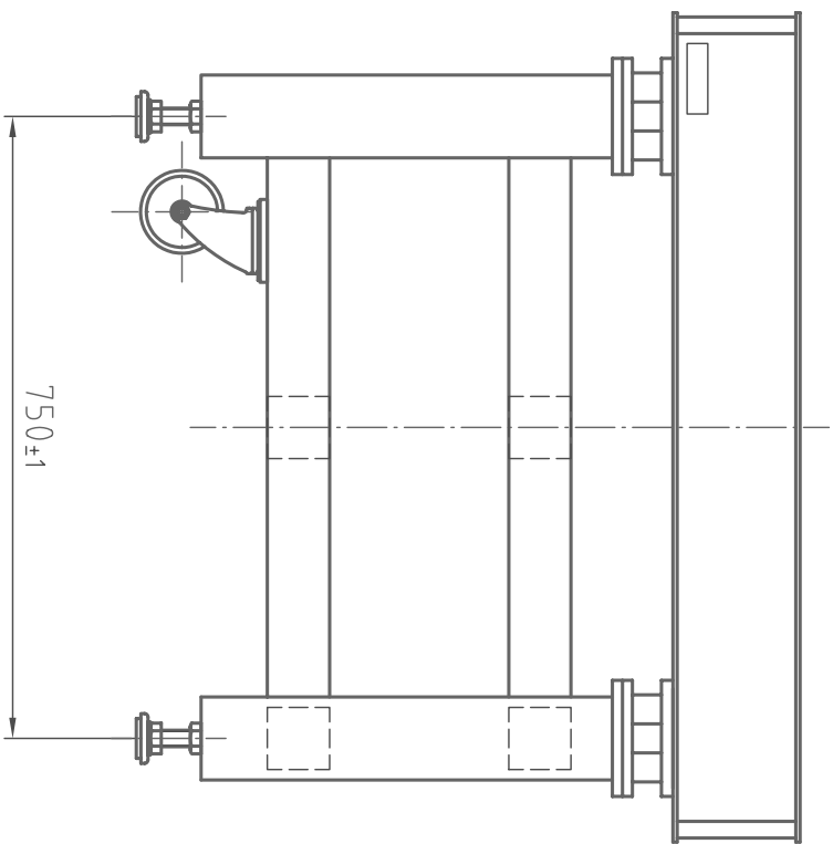
(右侧面图)
