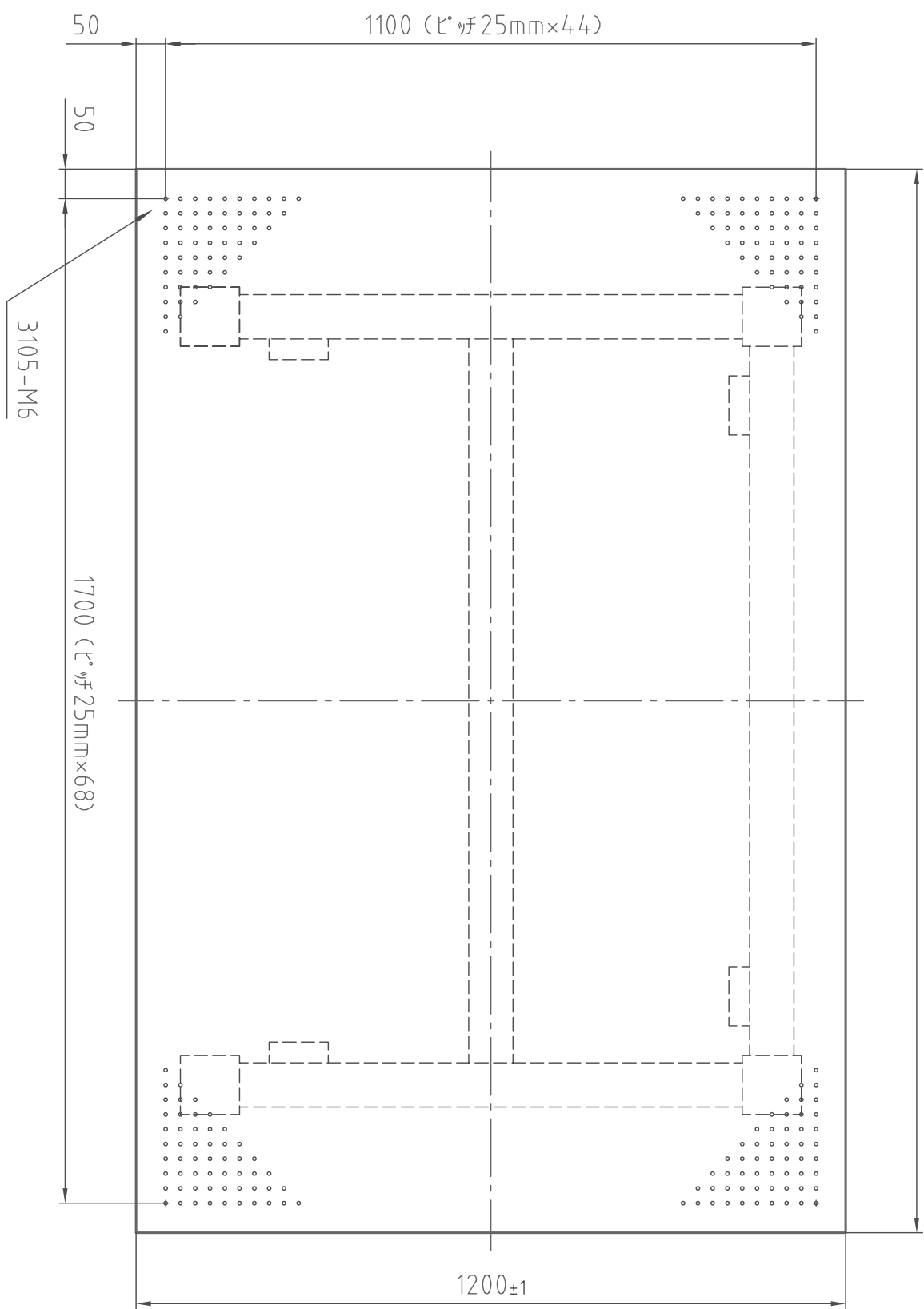
(平面図)
