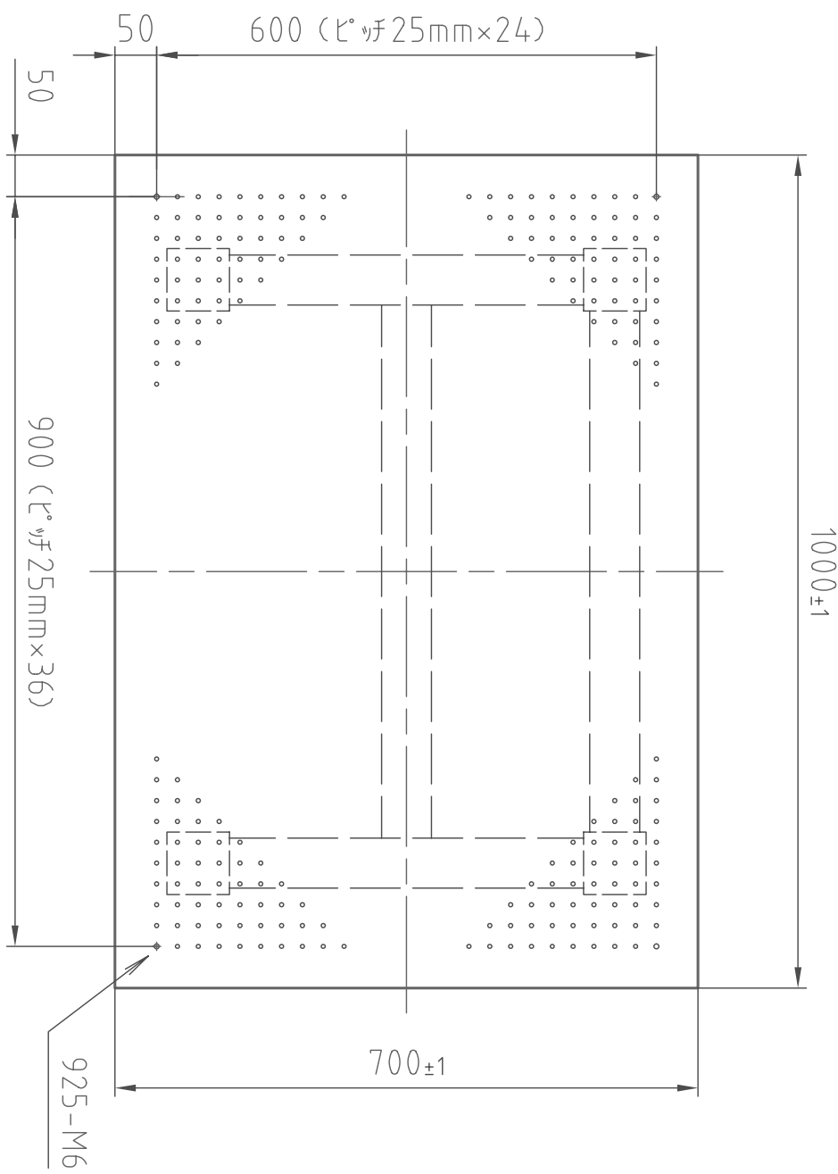
(平面図)
