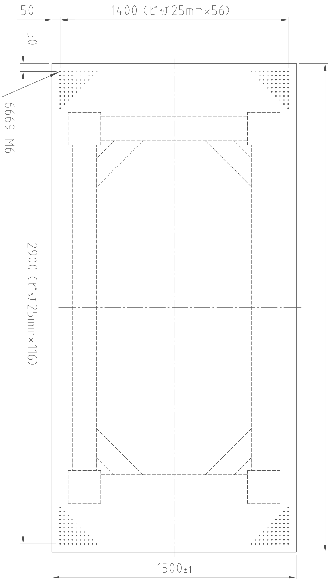
(平面図)
