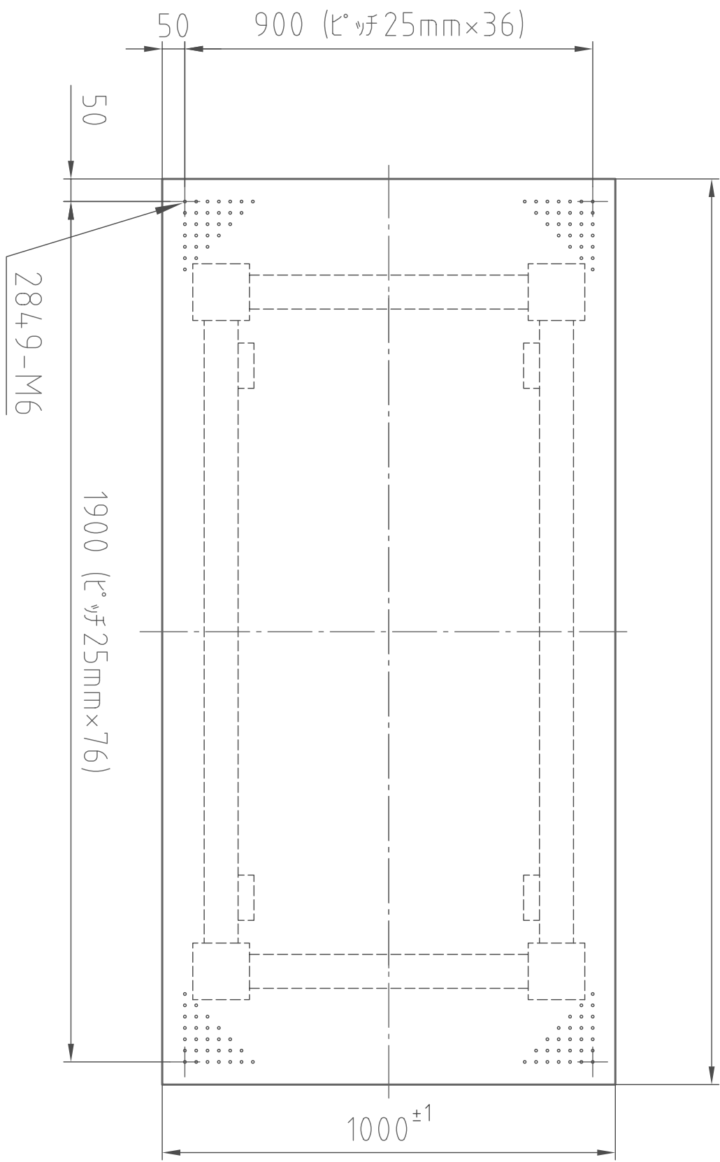
(平面図)
