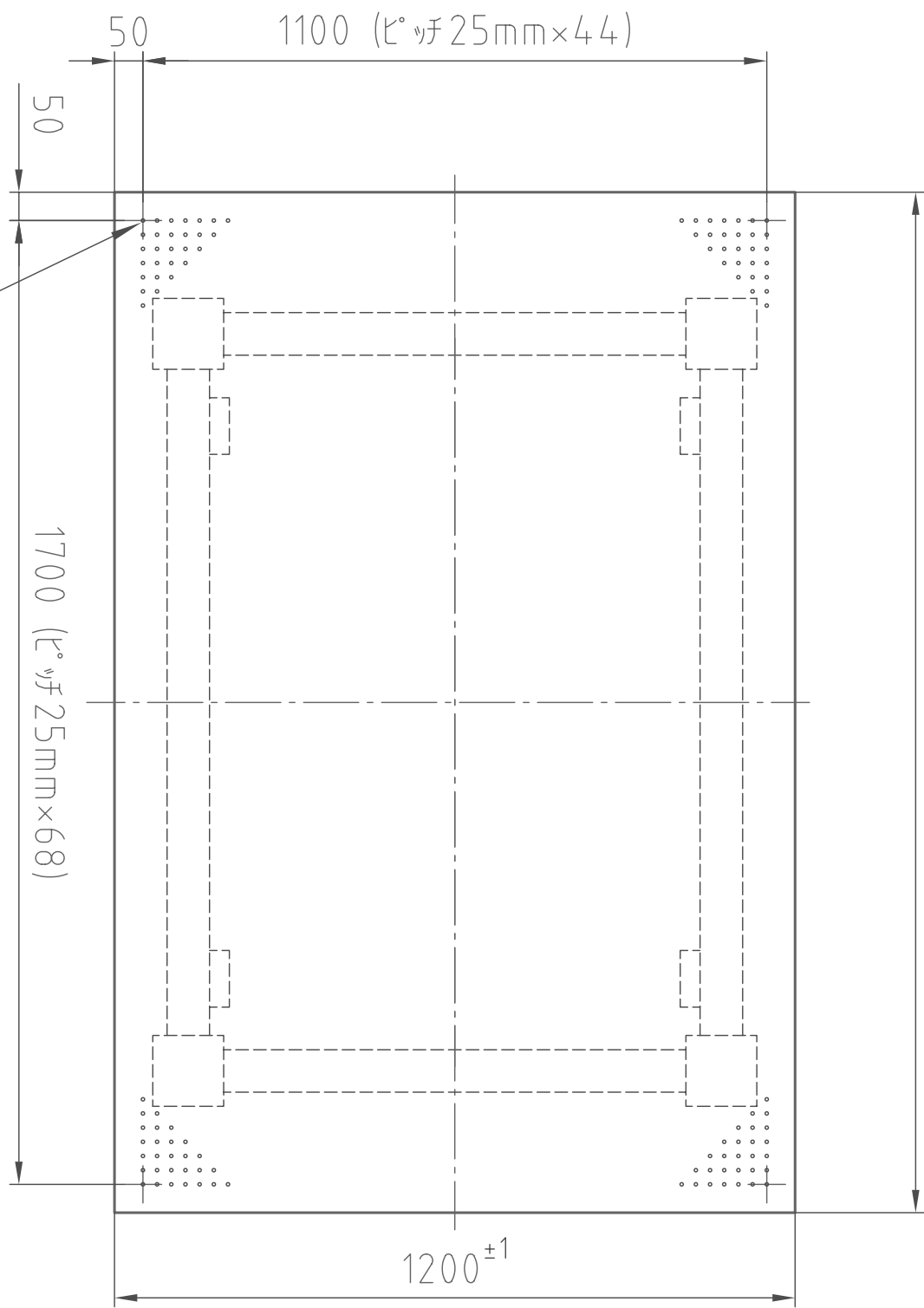
(平面図)
