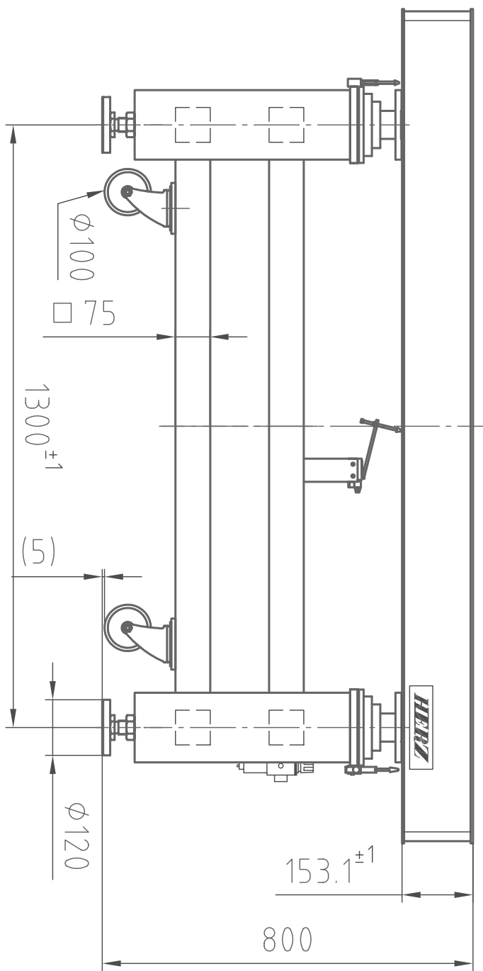
(正面図)
