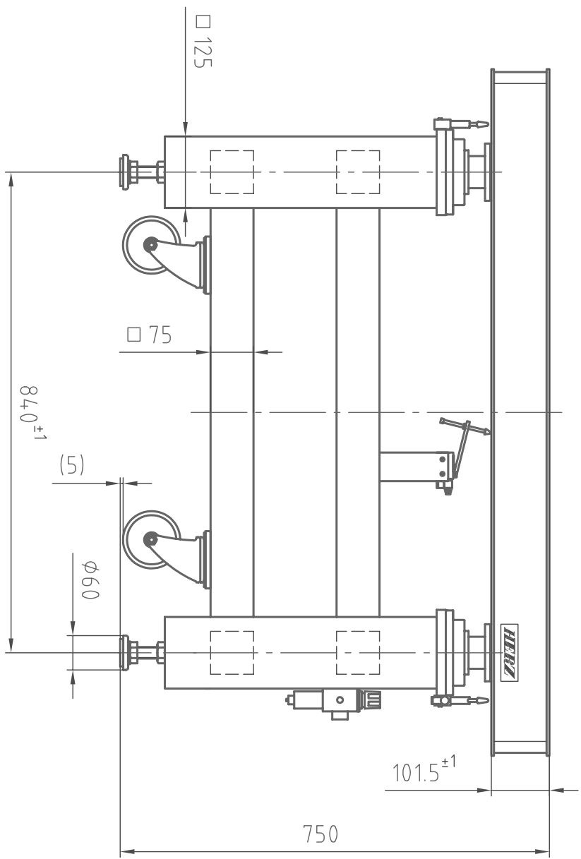
(正面図)
