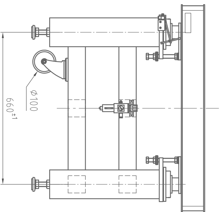
(右側面図)
