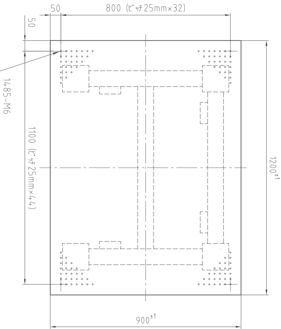
(平面図)
