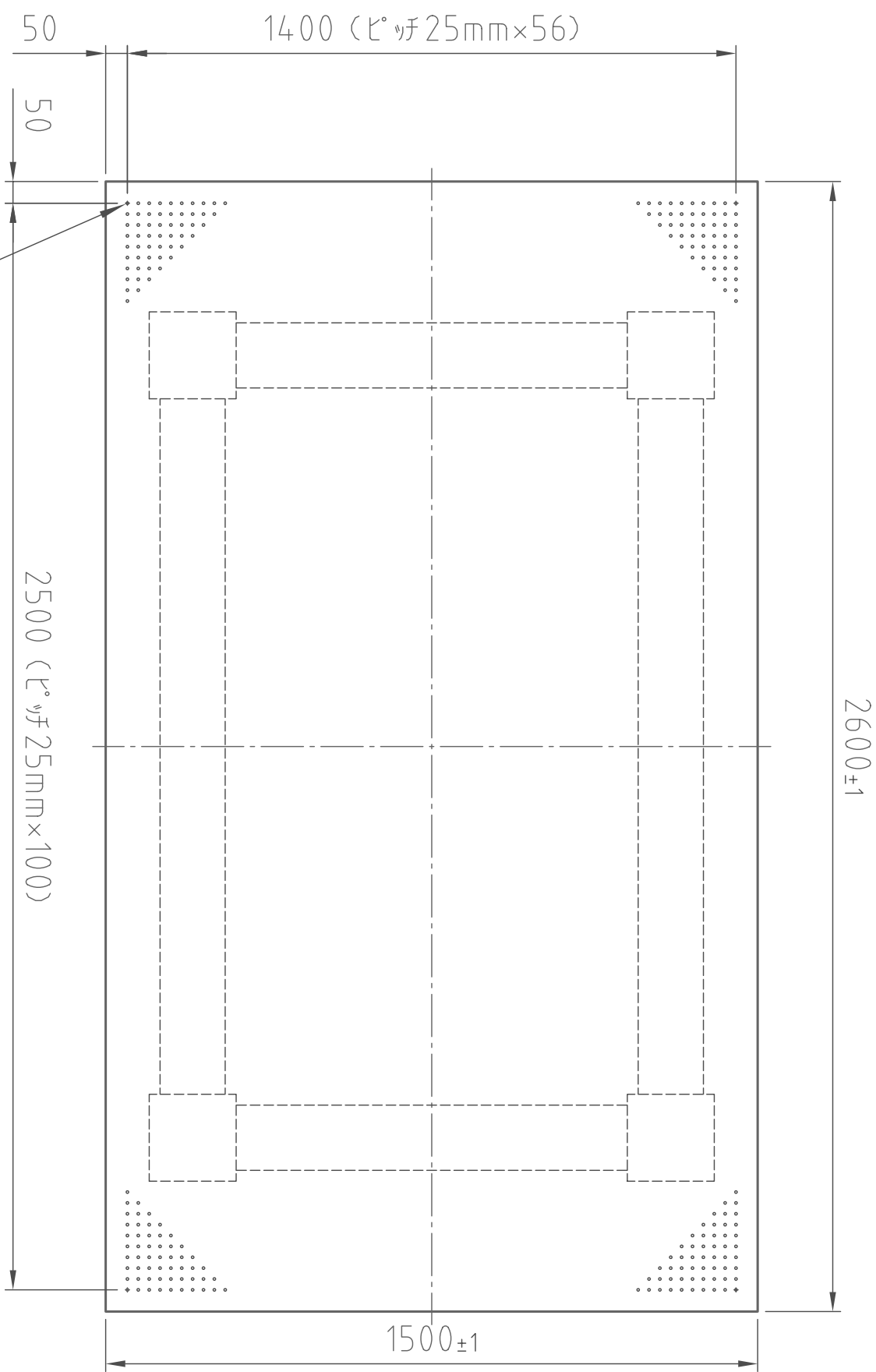
(平面図)
