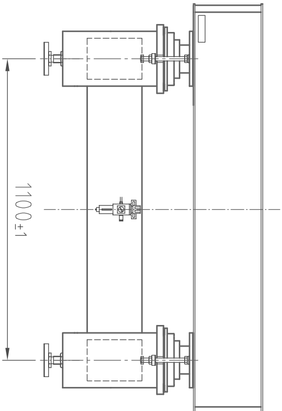
(右側面図)
