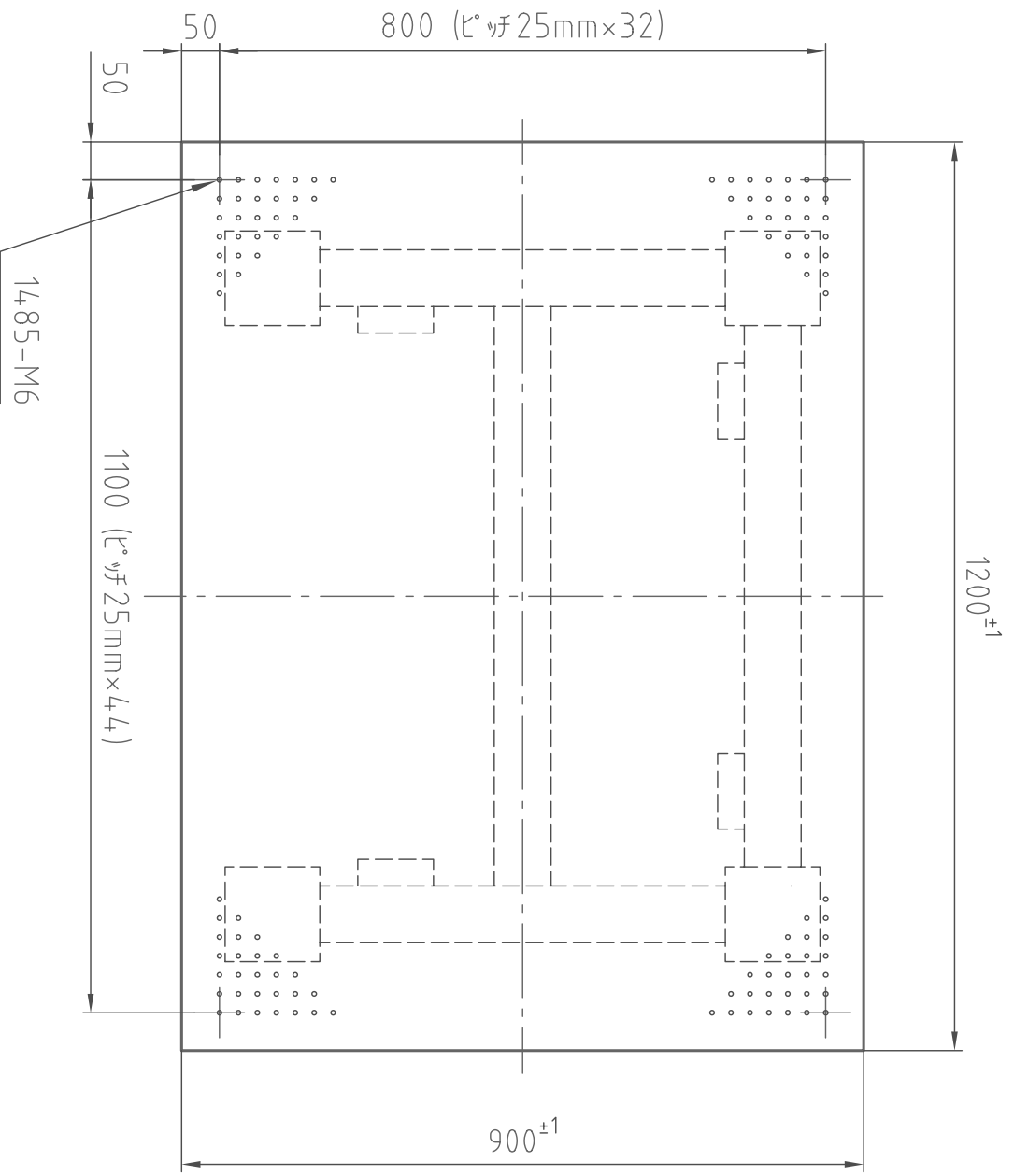
(平面図)
