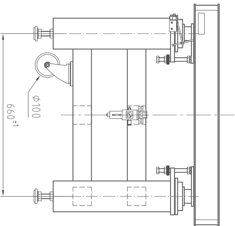
(右側面図)
