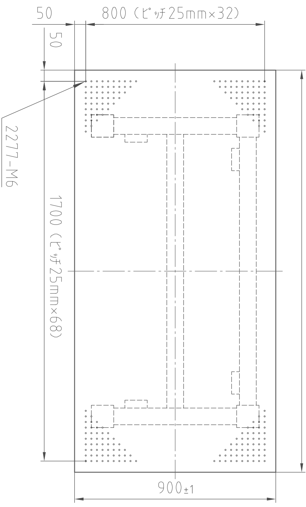
(平面図)
