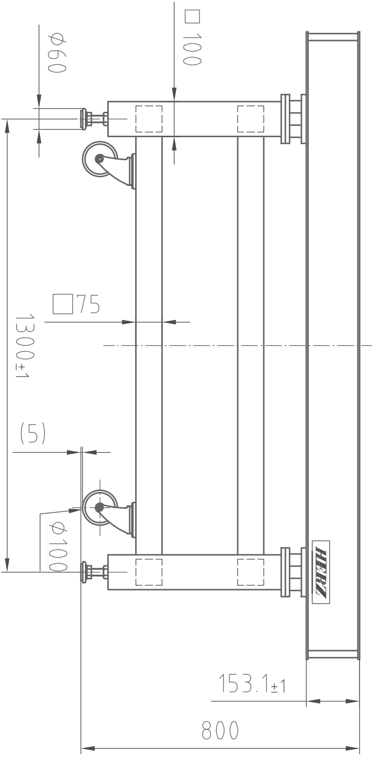
(正面図)
