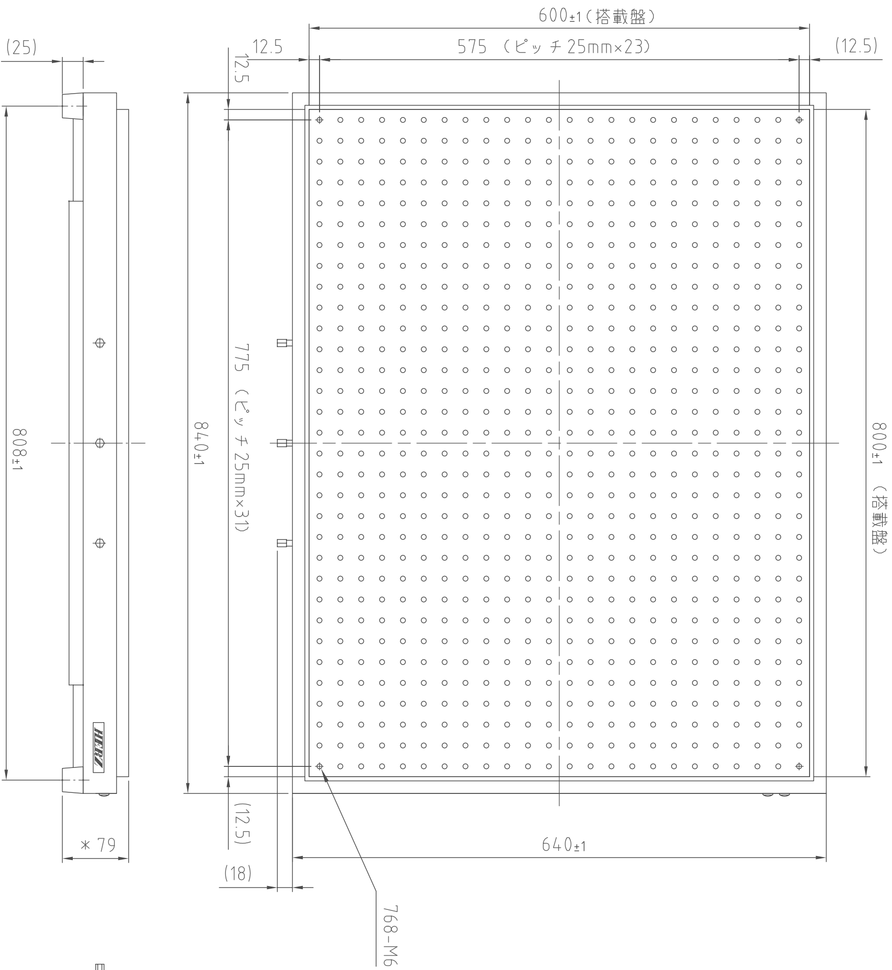
(正面図)
