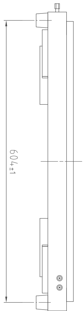
(右側面図)
