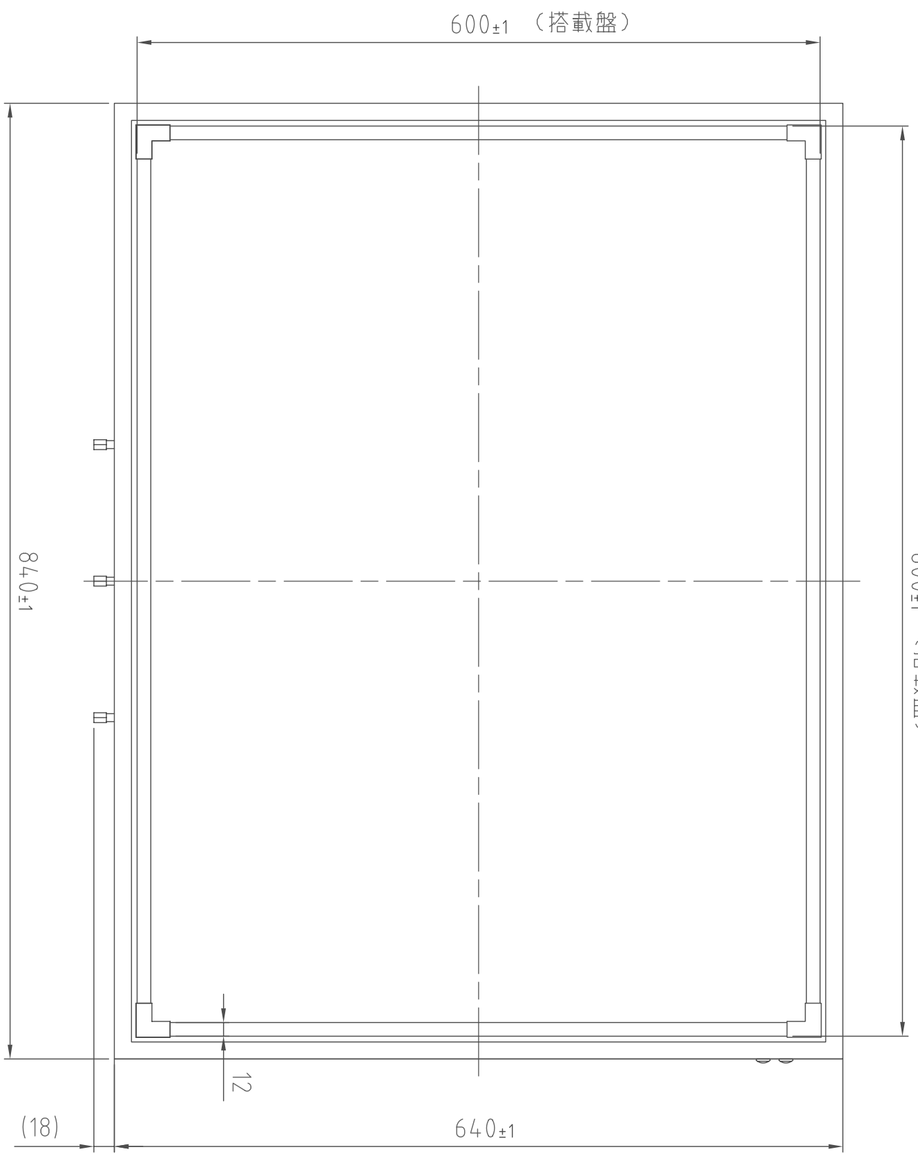
(平面図)
