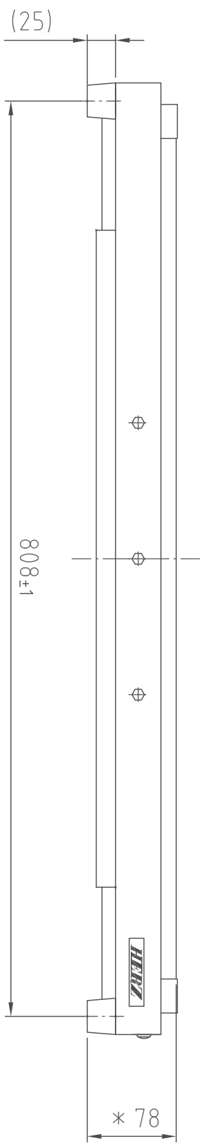
(正面図)
