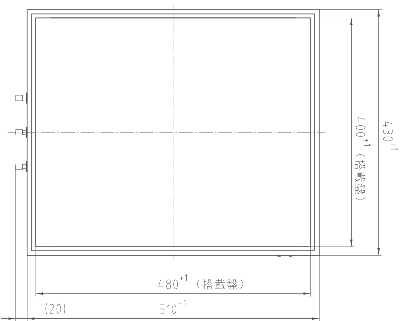
(平面図)
