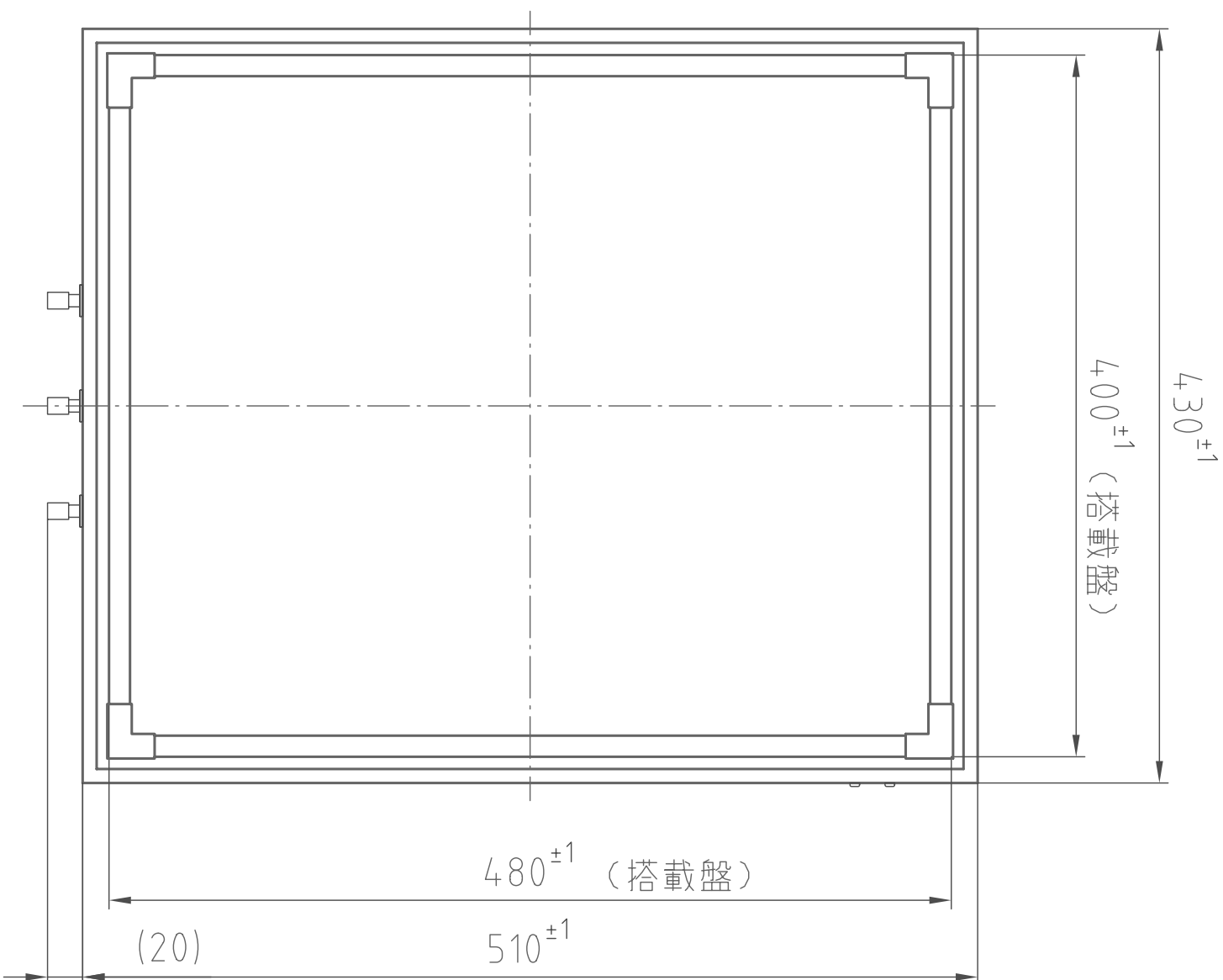
(平面图)
